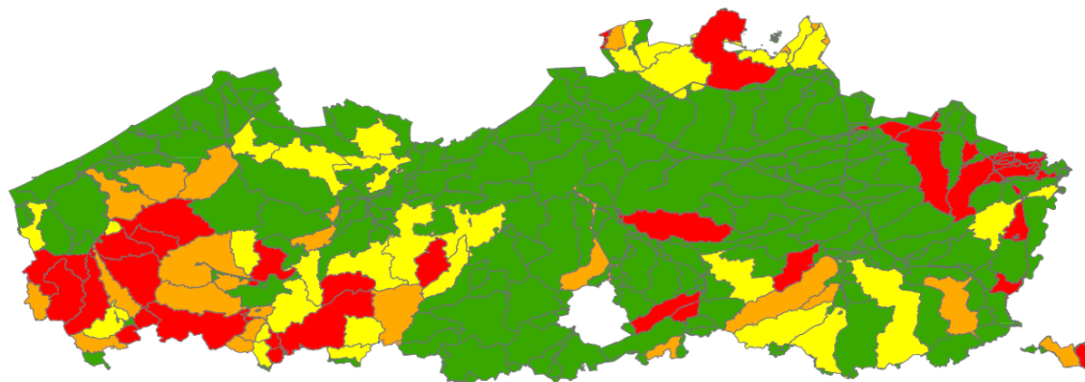
KAART 1B: EVALUATIE OPPERVLAKTEWATER - GEBIEDSTYPES
